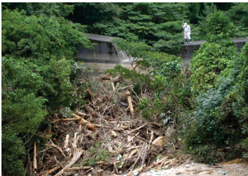
土や石を受け止めた さぼう 砂防えん てい 堤
