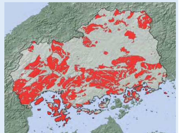
花崗岩類の分布
