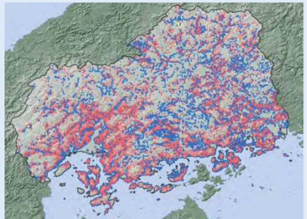
危険箇所の分布
